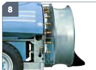
IT: Protezione contro l'aspirazione di corpi estranei / EN: Fan protection against leaves and soil remains / FR: Protection pour empêcher l'aspiration des feuilles / DE: Blätterschutz / ES: Protección contra la aspiración de hojas
